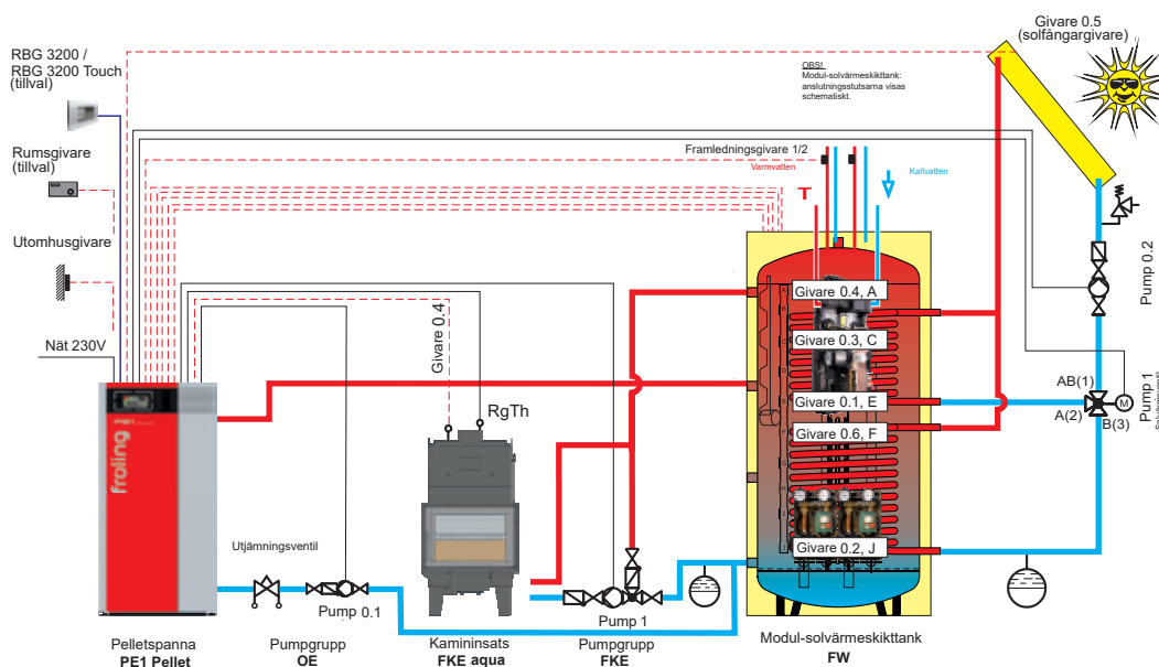
PE1 Pellet med tilläggsbränsla och modul-solvärmeskiktank FW
